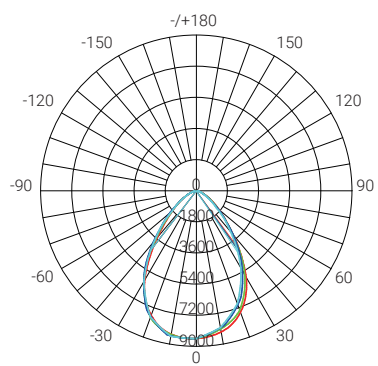
60° NEMA 4 - Medium
