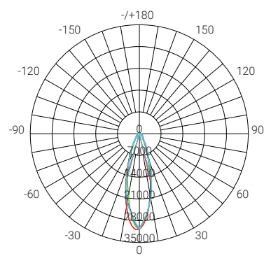
25° NEMA 3 - Narrow
