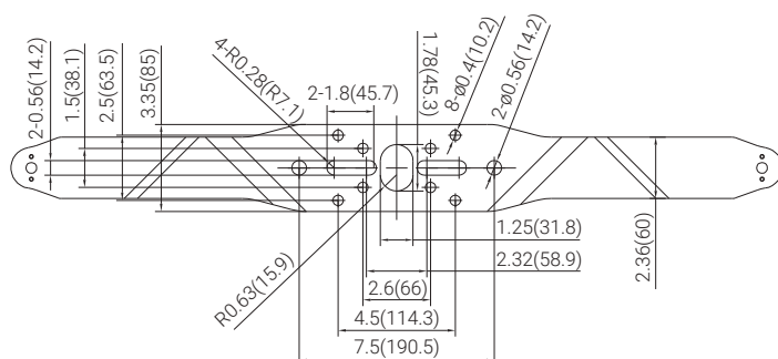
For 15L/20L/30L/40L
