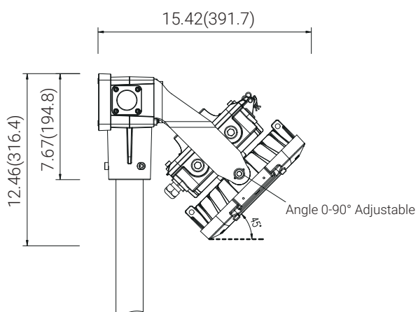
For 15L/20L/30L/40L
